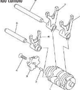
TAV.14 Comando cambio - Gear shift control - Commande changement de vitesse - Chaltung - Mando cambio
