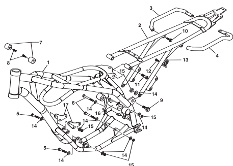
TAV.19 Telaio - Frame - Chassis - Rahmen - Chasis
