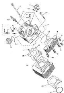
TAV.1 Cilindro - Cylinder - Cylindre - Zylinder - Cilindro
