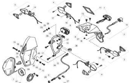
TAV.40B Impianto elettrico - Electrical equipment - Installation électrique - Elektrische anlage - Instalación electrica
