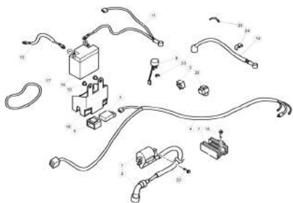
TAV.40A Dispositivi elettrici - Electrical devices - Dispositifs electriques - Elektrische Ausrüstung - Dispositivos electricos
