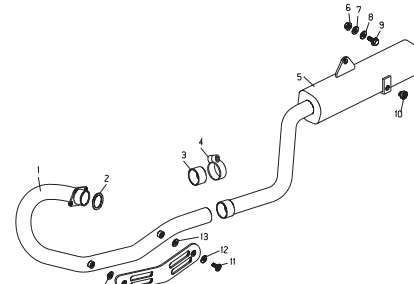
TAV.37 Marmitta - Silencer - Silencieux - Auspufftopf - Silenciador
