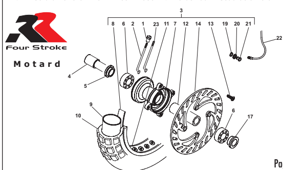
TAV.41 Ruota anteriore - Front wheel - Roue AV. - Vorderrad - Rueda delantera
