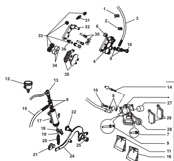
TAV.36 Impianto freno - Brake system - Circuit de freins - Bremsanlage - Instalació n frenos
