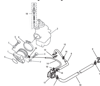
TAV.12 Carburatore-Raccordo d'ammissione - Carburettor-Induction pipe - Carburateur-Raccord d'admission - Vergaser-Ansaugstutzen - Carburador-Racor de admision
