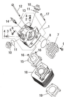
TAV.11A Cilindro - Cylinder - Cylindre - Zylinder - Cilindro
