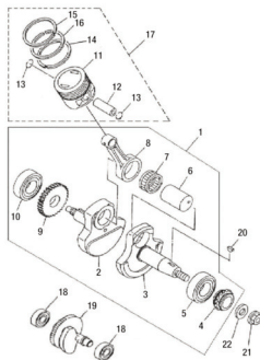
TAV.02 Albero motore-Pistone - Crankshaft-Piston - Vilebrequin-Piston - Kurbelwelle-Kolben - Cigüeñal-Pistó
