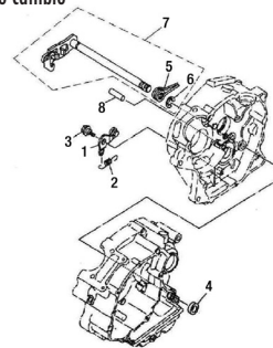
TAV.05A Comando cambio - Gear shift control - Commande changement de vitesse - Chaltung - Mando cambio
