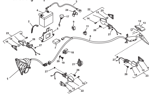
TAV.40A Dispositivi elettrici - Electrical devices - Dispositifs électriques - Elektrische Ausrüstung - Dispositivos eléctricos
