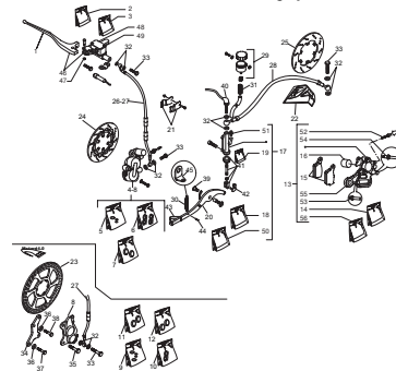
TAV.18 - Impianto frenante - Braking system
