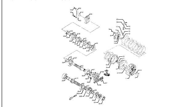
TAV.6 - Frizione - Clutch
