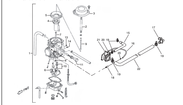
TAV.1 - Carburatore - Carburettor
