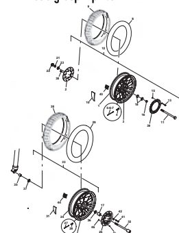
TAV.16 - Gruppo ruote - Wheels group Alp 4.0
