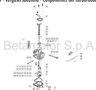
TAV.12B Componenti del carburatore - Carburettor component parts - Pieces composant le carburateur - Vergasersbauteile - Componentes del carburador
