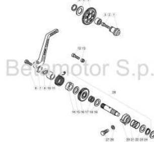
TAV.06 Avviamento a pedale - Kickstarter - Démarriage à pedal - Pedalstart - Arranque a pedal
