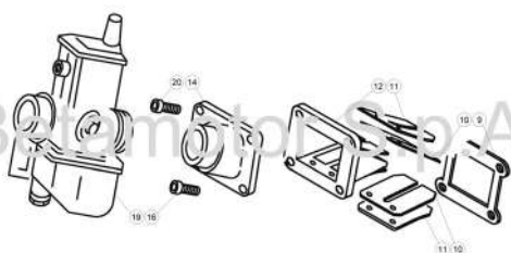
TAV.12A Carburatore - Carburettor - Carburateur - Vergaser - Carburador
