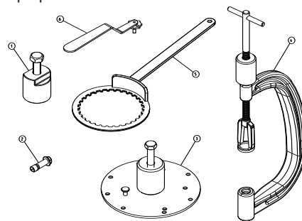
TAV.14 Attrezzatura specifica - Special tools - Outillage spécial - Spezialwerkzeug - Utillaje específico
