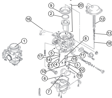
TAV.12 Carburatore - Carburettor - Carburateur - Vergaser - Carburador
