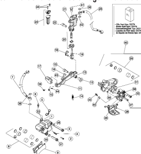
TAV.36 Impianto freni idraulici - Hydraulic brakes system - Installation des freins hydrauliques - Hydraulischebremseanlage - Instalación freno hidráulico
