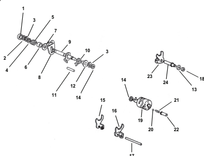
TAV.5 Comando cambio - Gear shift control - Commande changement de vitesse - Schaltung - Mando cambio
