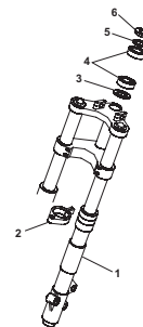
TAV.14 Forcella anteriore - Front fork - Fourche AV. - Vorderradgabel - Horquilla delantera
