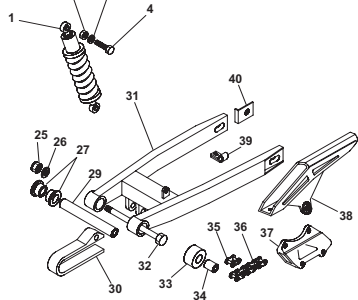
TAV.13 Sospensione posteriore - Rear suspension - Suspension AR. - Hintere aufhängung - Suspensión trasera
