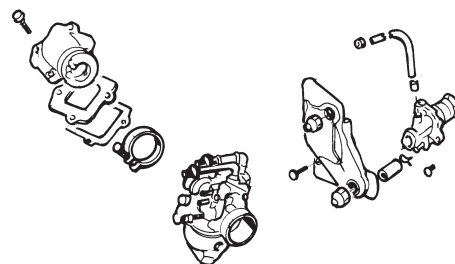
TAV.6 Pompa olio - Carburatore - Oil pump - Carburettor - Pompe huile - Carburateur - Ölpumpe - Vergaser - Bomba aceite - Carburador
