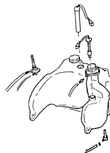
TAV.10 Serbatoio carburante-Serbatoio olio - Fuel tank-Oil tank - Reservoir carburant - Reservoir d'huile - Benzintank-Öltank - Tanque carburante-Deposito aceite
