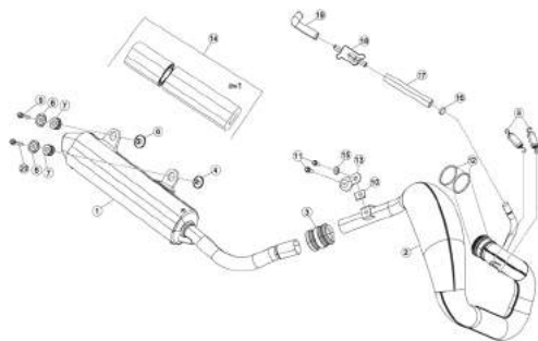
TAV.37A Gruppo scarico (omologato) - Exhaust system (homologated) - Echappement (homologué) - Auspuffanlage (homologierten) - Grupo escape (homologado)
