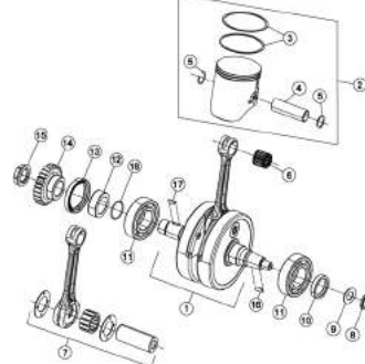
TAV.02 Albero motore - Crankshaft - Vilebrequin - Kurbelwelle - Cigüeñal
