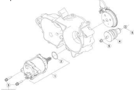
TAV.07 Avviamento elettrico - Electric starter - Dé marriage électrique - Elektrischer start - Arranque elétrico
