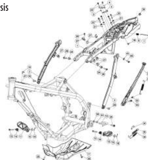
TAV.32 Accessori telaio - Frame accessories - Accessoires chassis - Rahmenzubehör - Accesorios Chasis
