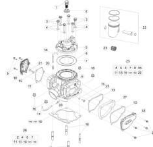
TAV.11 Cilindro completo - Cylinder, assy - Cylindre complet - Zylinder, KPL. - Cilindro completo
