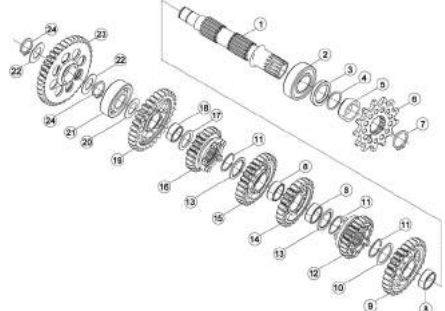
TAV.04B Albero secondario - Counter shaft - Arbre secondaire - Nebengetriebewelle - Eje secundario
