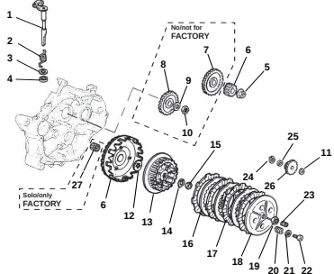
TAV.03 Gruppo frizione - Clutch unit - Groupe embrayage - Kupplung - Grupo embrague
