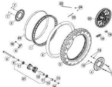
TAV.42 Ruota posteriore - Rear wheel - Roue AR. - Hinterrad - Rueda trasera (FACTORY - ENDURO - ENDURO STD)
