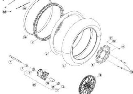
TAV.41 Ruota anteriore - Front wheel - Roue AV. - Vorderrad - Rueda delantera (TRACK)
