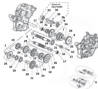
TAV.04 Gruppo ingranaggi cambio - Gear group - Engrenages changement de vitesses - Schaltgetriebe - Engranaje del cambio
