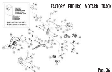
TAV.36 Impianto freni idraulici - Hydraulic brakes system - Installation des freins hydrauliques - Hidraulischebremse anlage - Instalació n freno hidráulico
