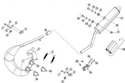
TAV.37 Gruppo scarico - Exhaust system - Echappement - Auspuffanlage - Grupo escape
