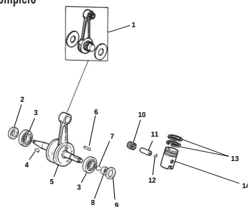
TAV.02 Gruppo imbiellaggio - Crankshaft assembly - Vilebrequin complet - Kurbelwelle Kpl. - Gr. bielas completo
