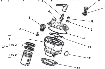
TAV.11 Gruppo cilindro-testa - Cylinder-cylinder head, assy - Esemble cylindre-culasse - Gruppe zylinder-Zylinderkopf - Grupo cilindro-culata
