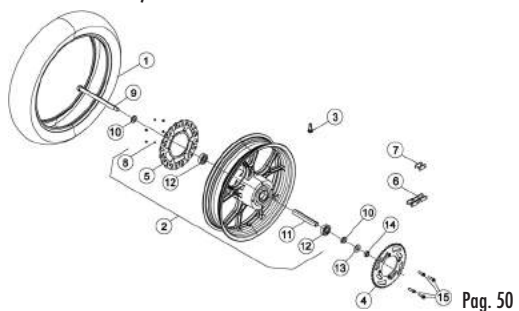
TAV.42 Ruota posteriore - Rear wheel - Roue AR. - Hinterrad - Rueda trasera (MOTARD - MOTARD STD)
