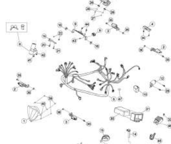
TAV.40 Impianto elettrico - Electrical equipment - Installation électrique - Elektrische anlage - Instalació n electrica
