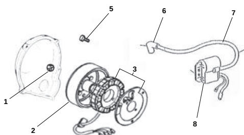
TAV.10 Gruppo accensione elettronica - Electronic ignition assy. - Groupe allumage électronique - Elektronischezündung gruppe - Grupo encendido electrónico
