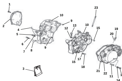
TAV.01 Basamento - Crankcase - Carter - Kurbelgehäuse - Carter
