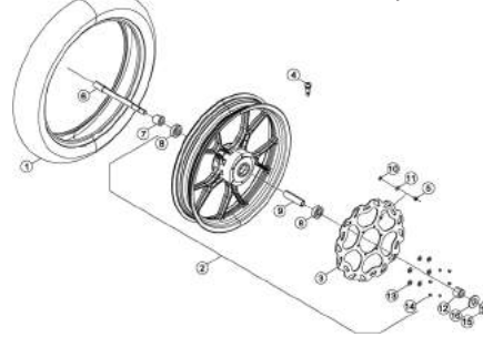
TAV.41 Ruota anteriore - Front wheel - Roue AV. - Vorderrad - Rueda delantera (MOTARD - MOTARD STD)
