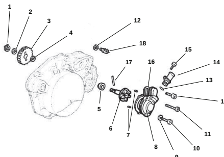
TAV.09 Impianto di raffreddamento - Installation de refroidissement - Installation de refroidissement - Kühlsystem - Instalación de enfriamiento
