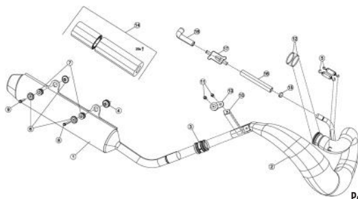
TAV.37A Gruppo scarico (omologato) - Exhaust system (homologated) - Echappement (homologué) - Auspuffanlage (homologierten) - Grupo escape (homologado)
