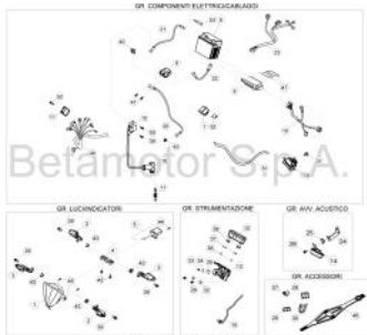
TAV.40 Impianto elettrico - Electrical equipment - Installation électrique - Elektrische anlage - Instalaci3n electrica
