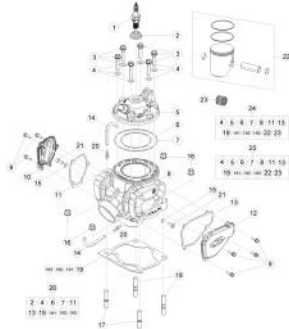
TAV.11 Cilindro completo - Cylinder, assy - Cylindre complet - Zylinder, KPL - Cilindro completo
