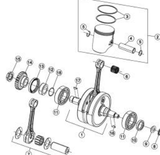
TAV.02 Albero motore - Crankshaft - Vilebrequin - Kurbelwelle - Cigüeñal
