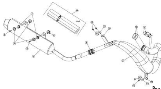
TAV.37B Gruppo scarico (gara) - Exhaust system (race) - Echappement (course) - Auspuffanlage (rennen) - Grupo escape (carrera)
