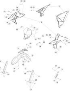
TAV.43A Carenature-Parafanghi - Mudguards - Carenages-Gardeboues - Verkleidungen-Kotflügel - Carenados-Guardabarros
