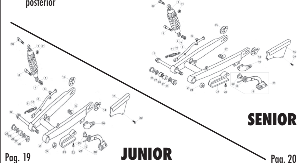
TAV.33 Forcellone posteriore - Rear fork - Fourche arriere - Hinterradschwinge - Horquilla posterior
