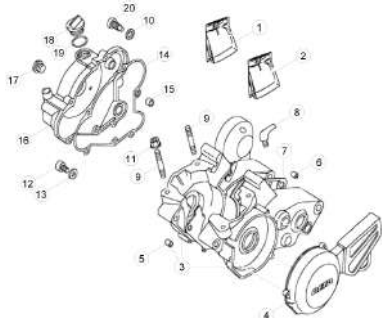
TAV.01 Basamento - Crankcase - Carter - Kurbelgehäuse - Carter
