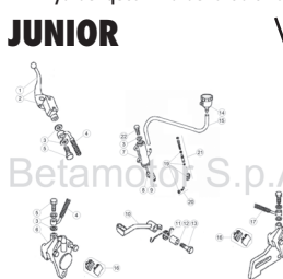
TAV.36 Impianto freni idraulici - Hydraulic brakes system - Installation des freins hydrauliques - Hidraulischebremse anlage - Instalació n freno hidráulico
