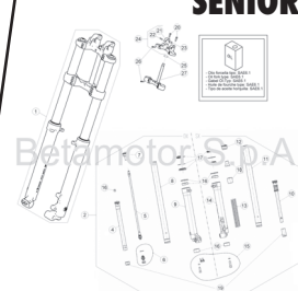
TAV.34 Forcella anteriore - Front fork - Fourche AV - Vorderradgabel - Horquilla delantera
