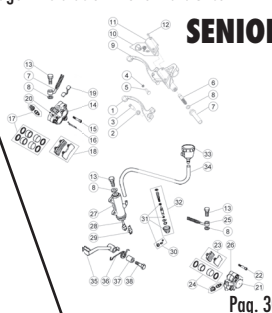
TAV.36 Impianto freni idraulici - Hydraulic brakes system - Installation des freins hydrauliques - Hidraulischebremse anlage - Instalació n freno hidráulico
