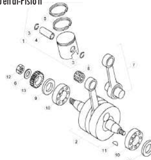
TAV.02 Albero motore-Pistone - Crankshaft-Piston - Vilebrequin-Piston - Kurbelwelle-Kolben - Cigüeñal-Pistón
