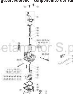
TAV.12B Componenti del carburatore - Carburettor component parts - Pieces composant le carburateur - Vergasersbauteile - Componentes del carburador
